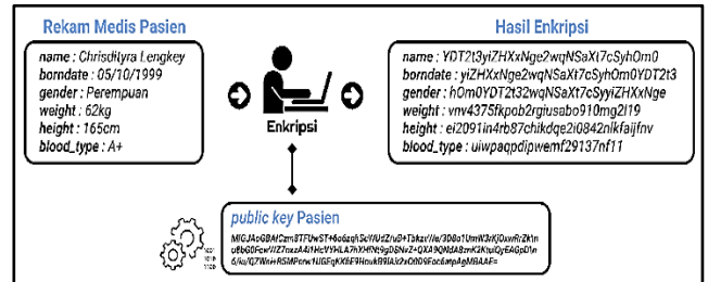
Gambar 9. Alur Enkripsi
