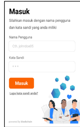
Gambar 23 Login
